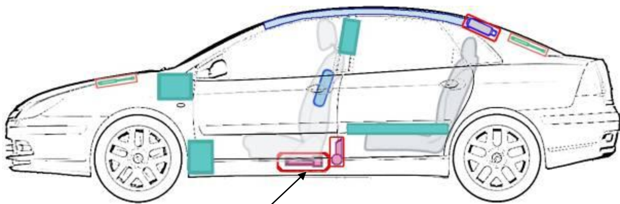
Pyrotechnischer Gurtstraffer auf Beifahrerseite vorne (Lage hinter der B-Säule)
