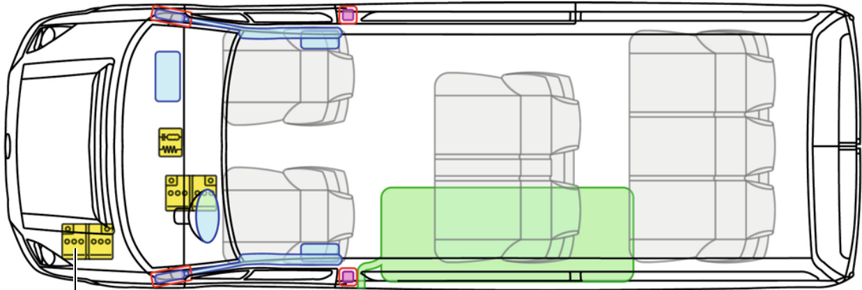
ausstattungsabhängig 2. Batterie im Motorraum
